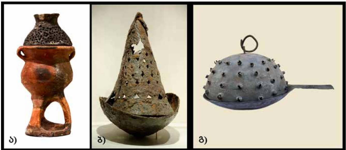
6. საქართველოს ტერიტორიაზე აღმოჩენილი და თეოფილუსის მიერ აღწერილი მუფელები: ა). ურბნისში, ტვლეპია გორაზე, ქვაცხელაში აღმოჩენილი თიხის მუფელი. ძვ.წ. IV ათასწლეულის დასასრული – III ათასწლეულის დასაწყისი; ბ). ვანის ნაქალაქარში აღმოჩენილი რკინის მუფელი – კოლხური ხუფი. ძვ.წ. I ს.; გ). თეოფილუსის (XI ს.) მიერ აღწერილი რკინის მუფელი (რეკონსტრუირებულია ერ. მაღრაძის მიერ) Muffles found in the territory of Georgia and described by Theophilus: a) clay muffle found on Kvatskhela on Telepia hill in Urbnisi. End of the IV millennium – beginning of the III millennium; b) iron muffle-Colchian cover-found on Vani site of former settlement. 1 st c. BC. c) iron muffle described by Theophilus – 11 th c. (reconstructed by Er. Magradze)
