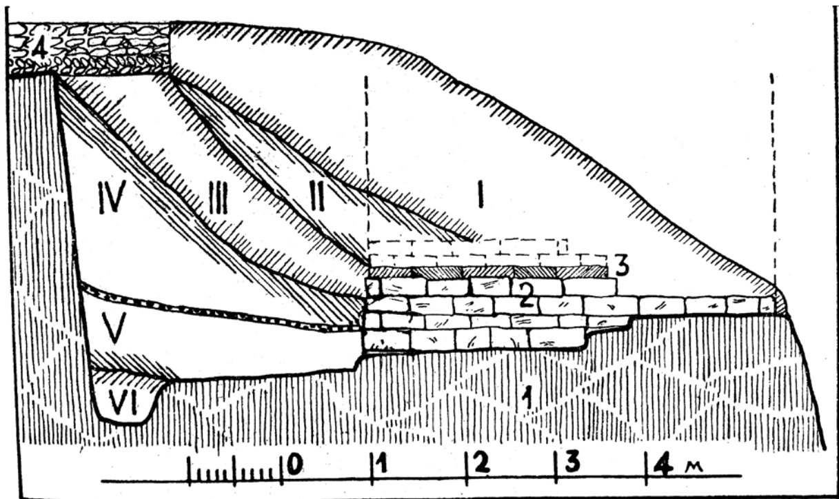
2 შიდა ქალაქი. ფენების განლაგების სქემატური ჭრილი Inner Town. District II. Schematic section of layer arrangement
