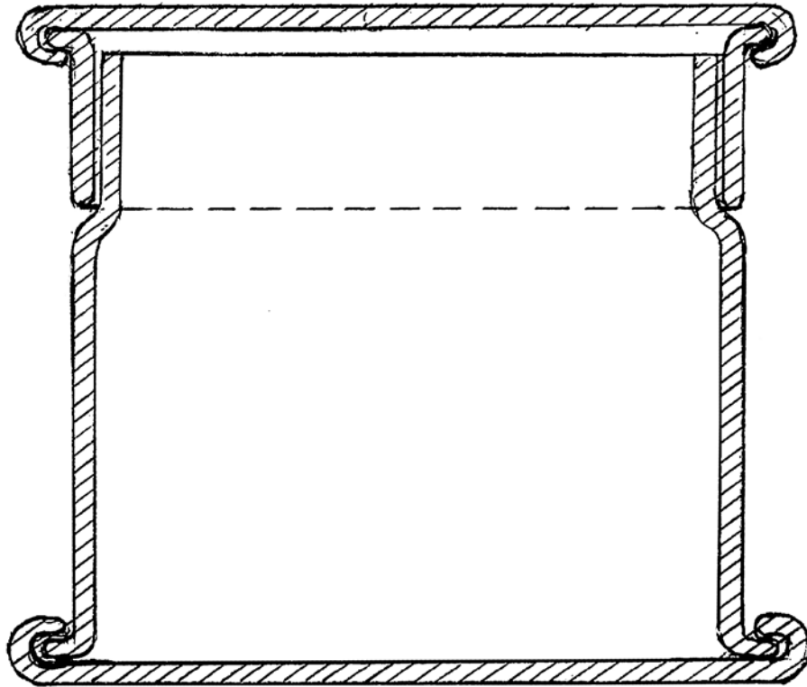
5. უფლისციხის შიდა ქალაქის რკინის მუფელის ნახაზი (შესრულებულია ერ. მაღრაძის მიერ) Drawing of an iron muffle of the inner town of Uplistsikhe (made by Er. Magradze)
