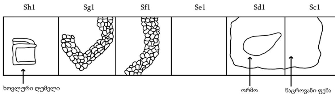
თხრილი N1. Sc1/Sh1 კვადრატების გეგმა Trench 1. Plan of Sc1-Sh1 squares
